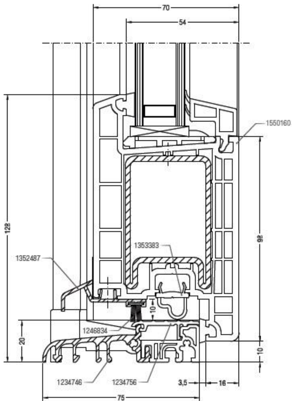
Sezione nodo anta dritta da 98 mm e soglia in Al Brillant 70
